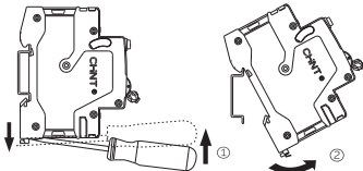
TH35-7.5 DIN Rail
