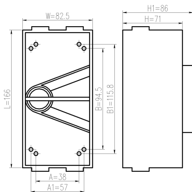
图A1 外形尺寸及安装尺寸
