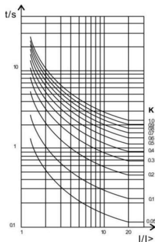
IDMT Normal Inverse
